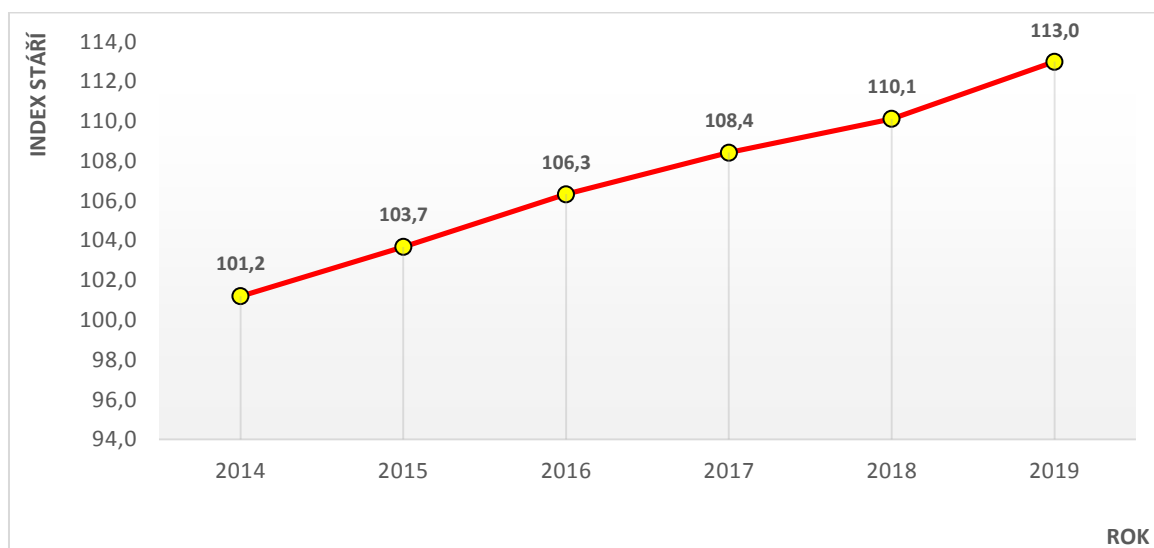
Graf 3 Vývoj indexu stáří v regionu MAS Hradecký venkov v letech 2014–2019
