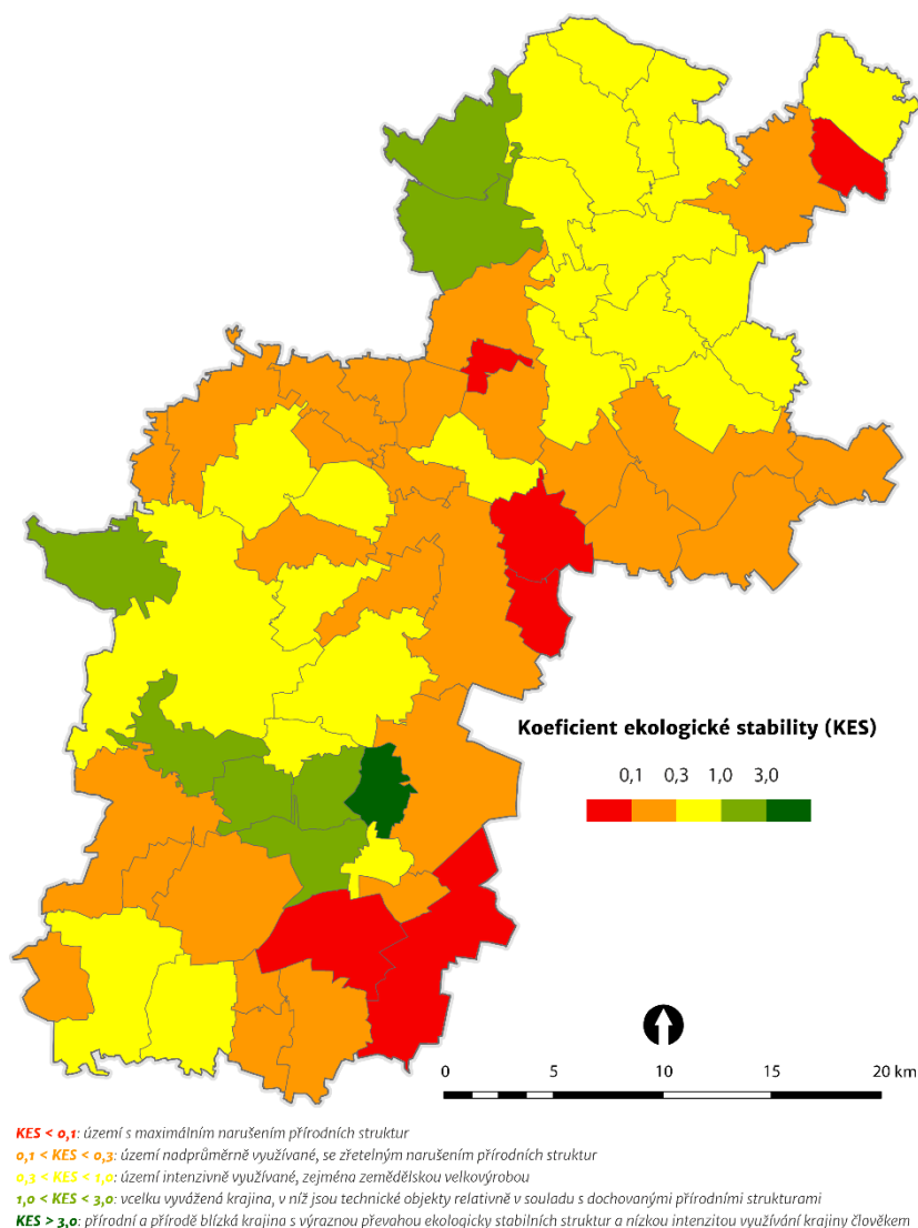
Obrázek 17 Koeficient ekologické stability v obcích MAS Hradecký venkov v roce 2019
