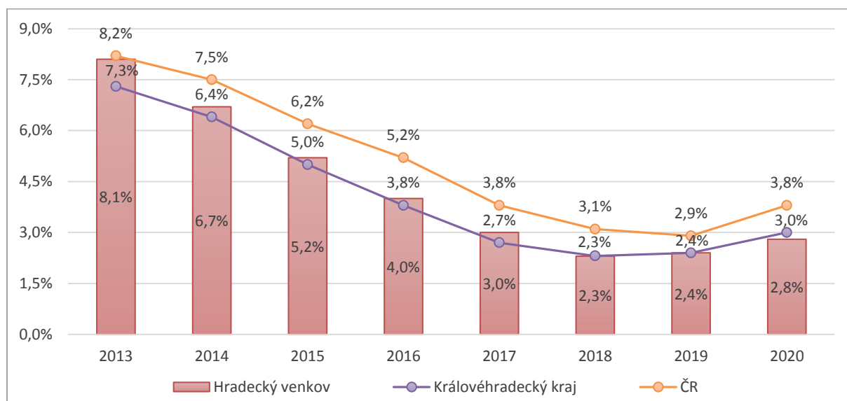
Graf 9 Vývoj podílu nezaměstnaných osob v území Hradeckého venkova v letech 2013–2020
